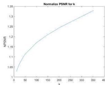
(b) NPSNR
