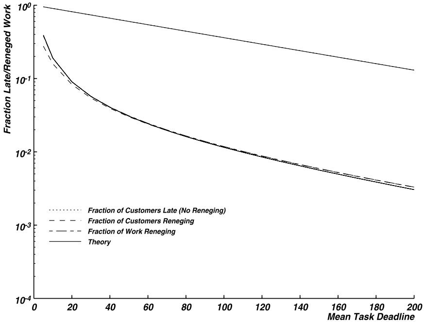
FIG. 1. M/M/1 queue.
