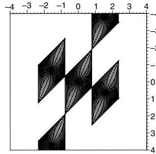
(d) Projection of (c) onto xy -plane
