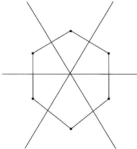
FIG. 4. The zonotope Z .
