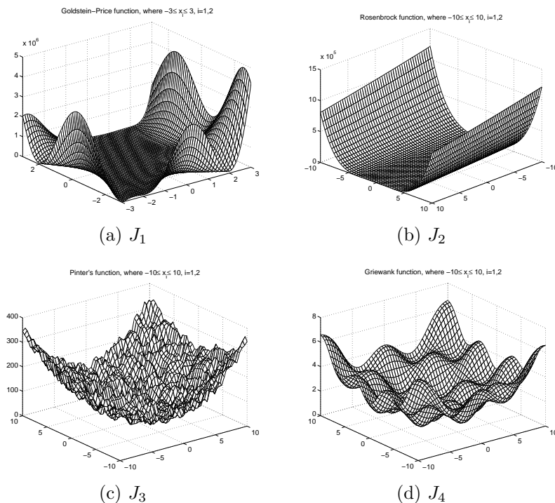
FIG. 2. Test functions (deterministic version) in two dimensions, (a) J_1 : Goldstein-Price; (b) J_2 : Rosenbrock; (c) J_3 : Pinter; (d) J_4 : Griewank.
