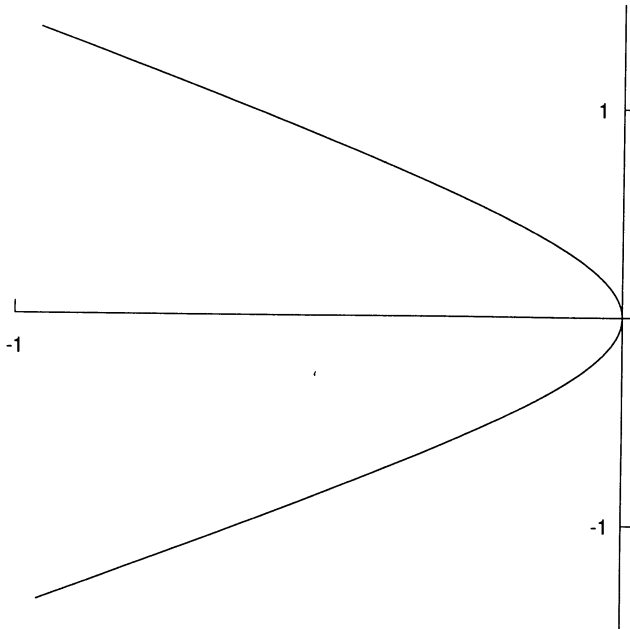
FIG. 1. The parameter space \Theta .
